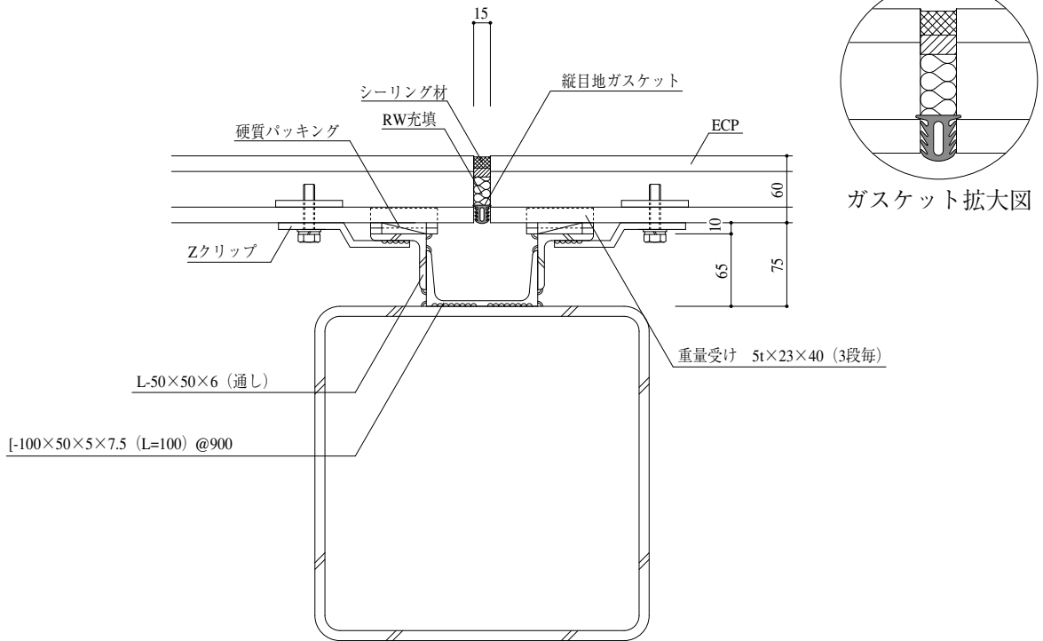
水平断面図
