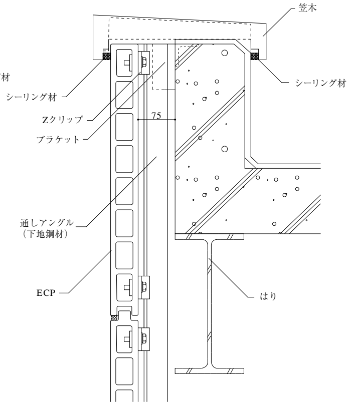
図4-11 横張り工法上部標準詳細図
