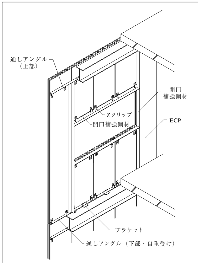
図1-1 縦張り工法
