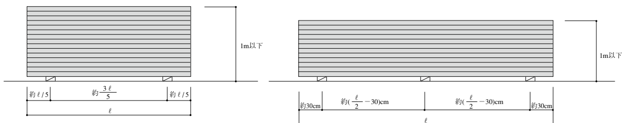
パネル長さが4m以下の場合
