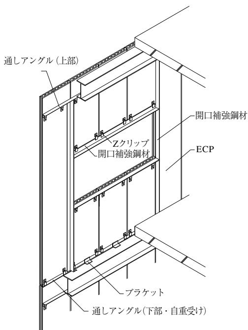
図4-1 縦張り工法
