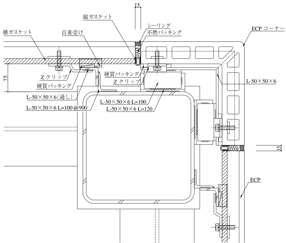
出隅コーナー部詳細図
