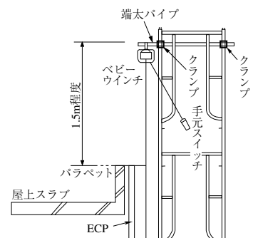
図3-3 足場
