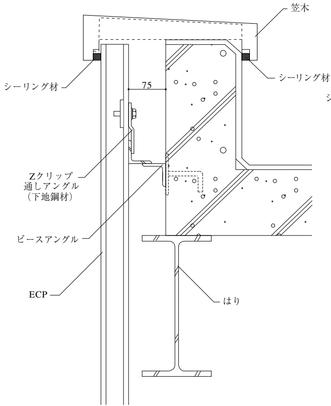
図4-10 縦張り工法上部標準詳細図
