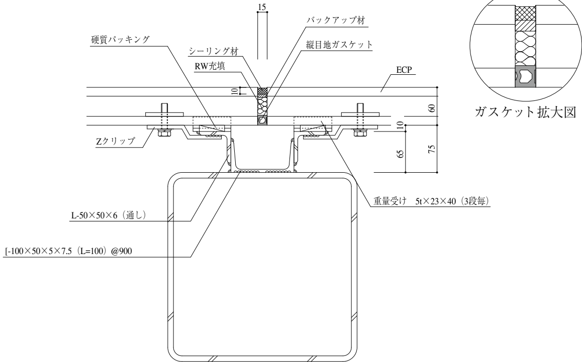
水平断面図
