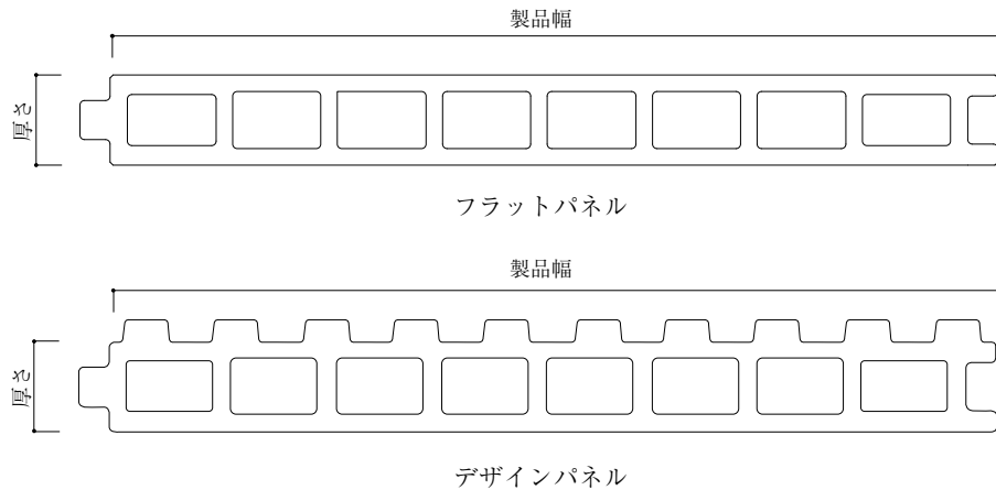
図2-2 形状の例
