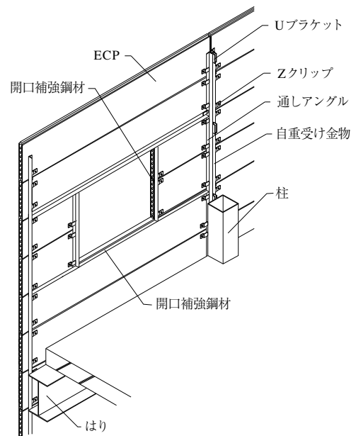
図4-2 横張り工法
