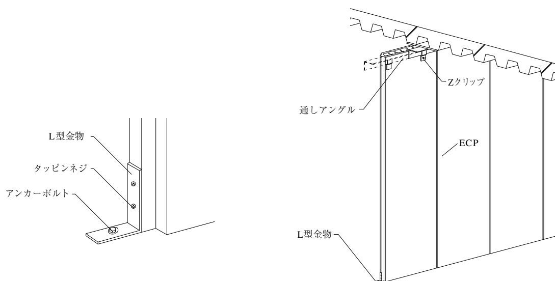
図5-1 L型金物工法
