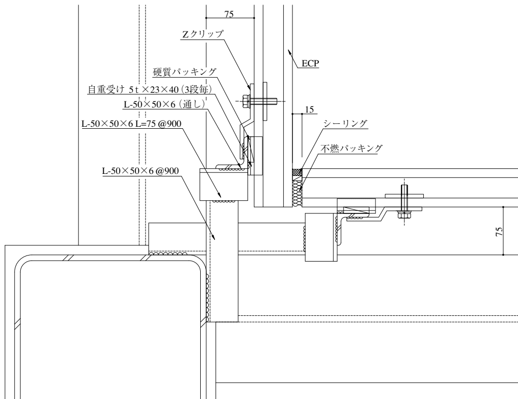
1-12 入隅コーナー部詳細図
