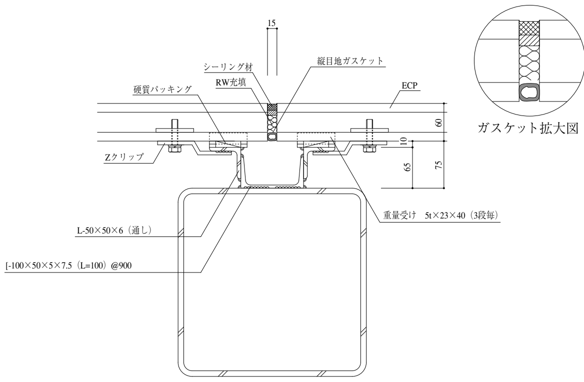
水平断面図
