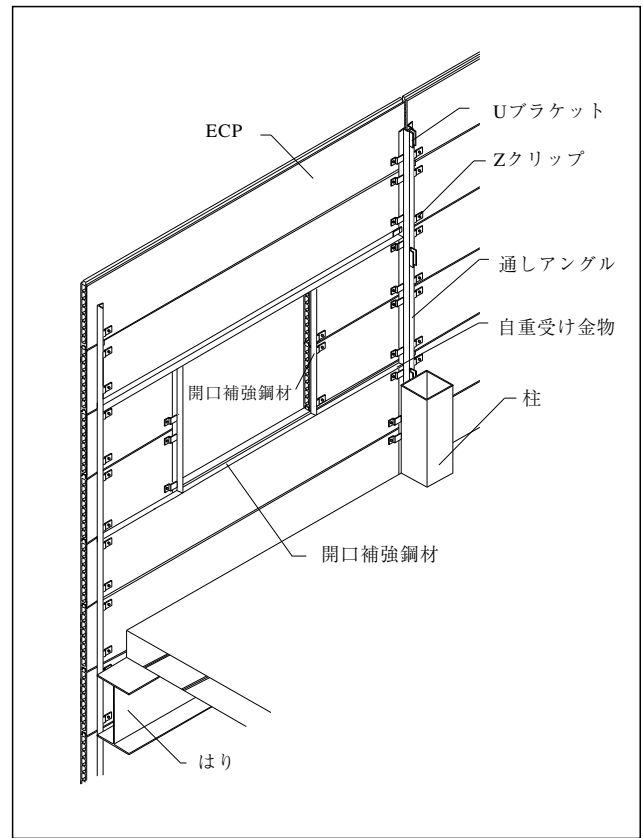
図1-2 横張り工法
