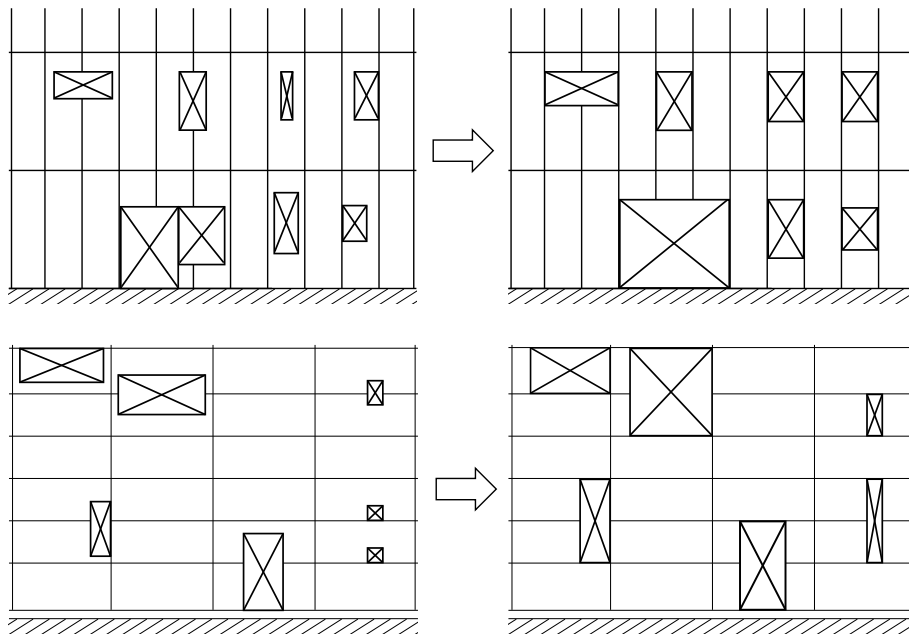
図3-6 パネル割付けの良否例
