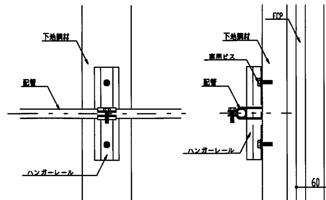
縦張り工法 ハンガーレール
