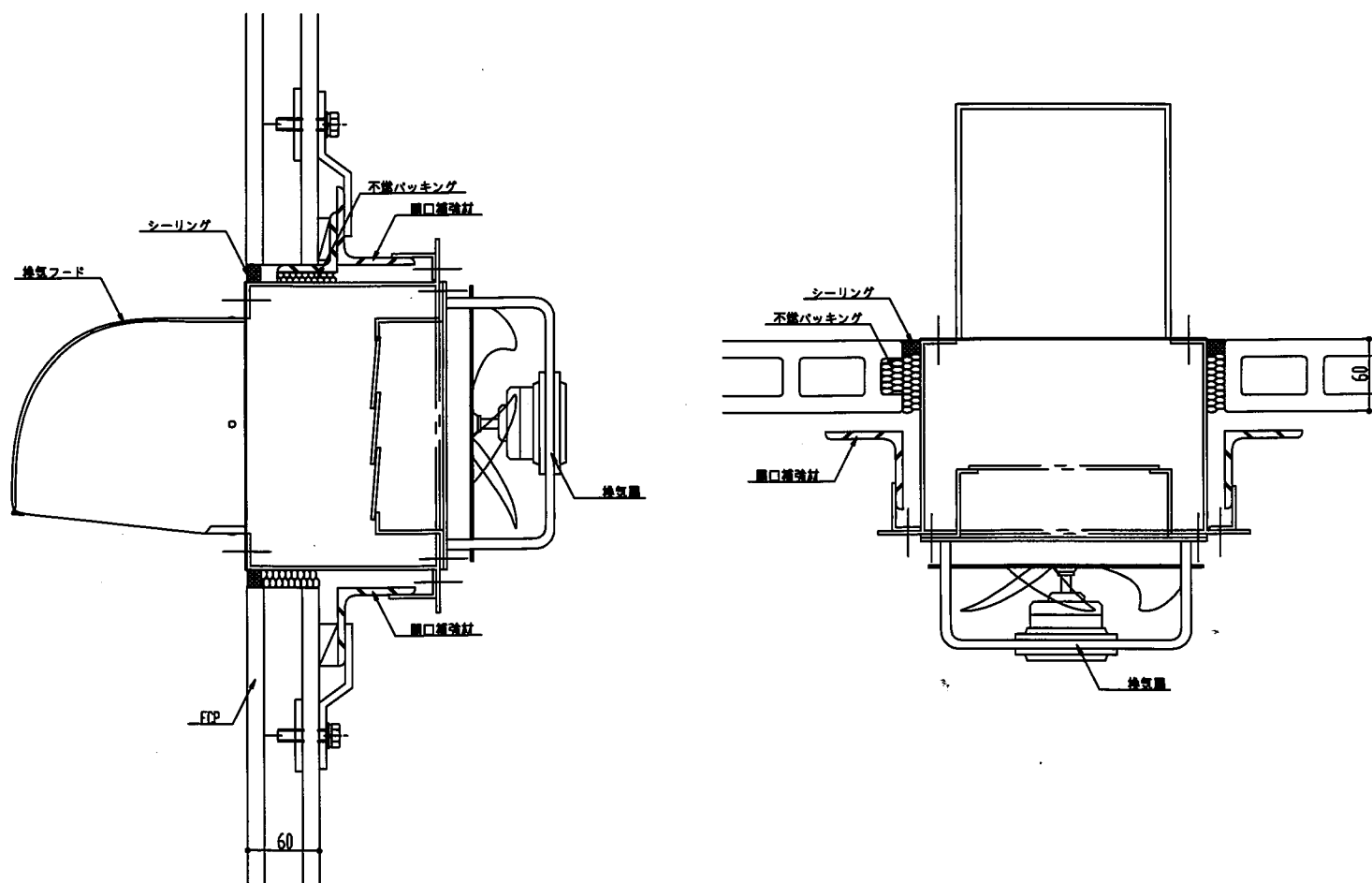
縦張り工法 換気扇
