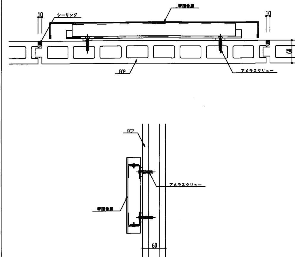
縦張り工法 サドル（サドルベース）
