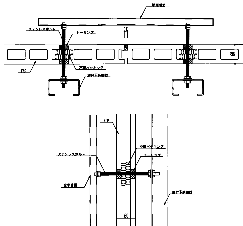
縦張り工法 ハンガーレール
