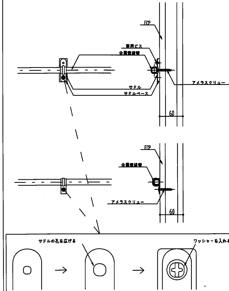
縦張り工法 サドル（サドルベース）
