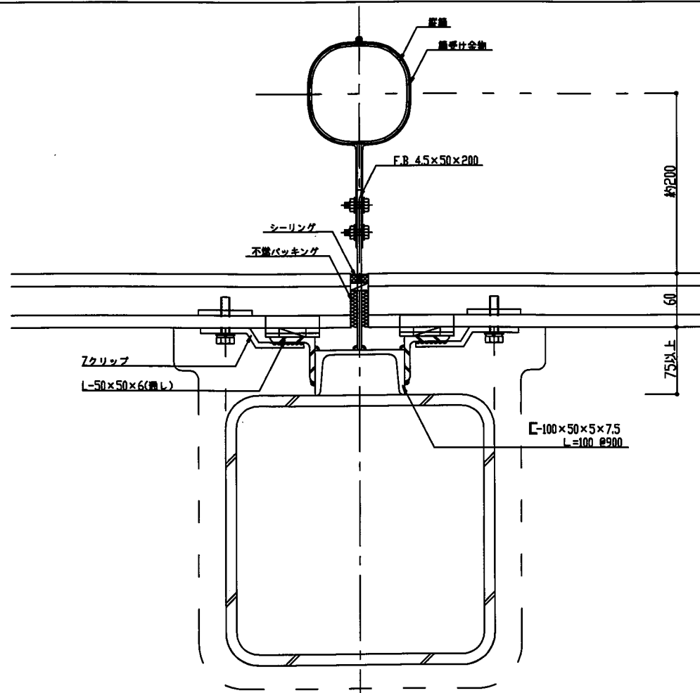
横張り工法 桶取合い
