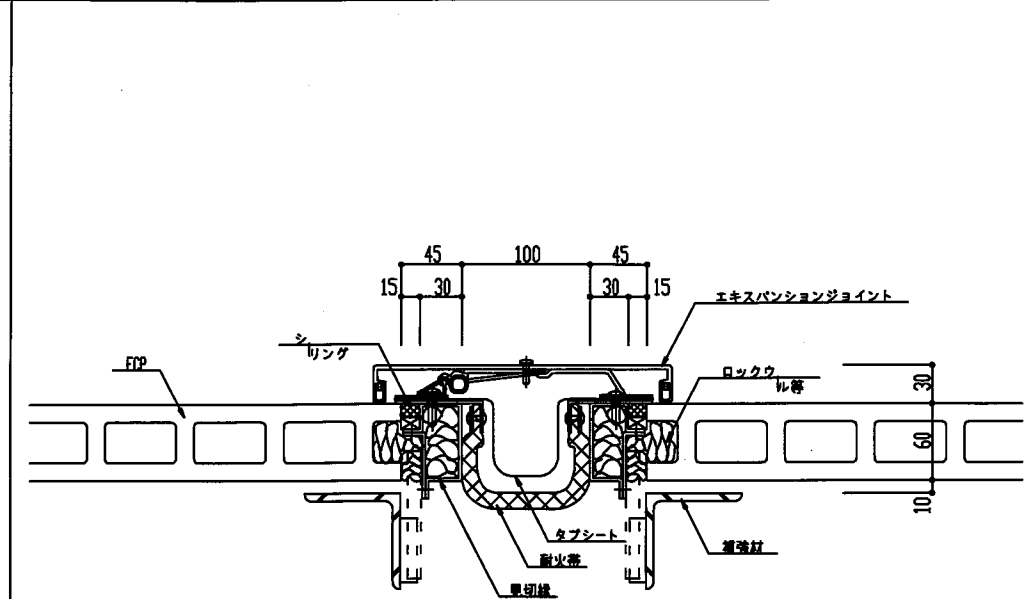
縦張り工法 エキスパンション取合い
