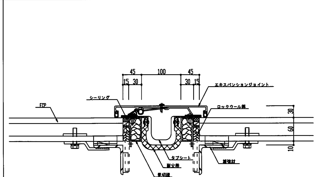
横張り工法 エキスパンション取合い
