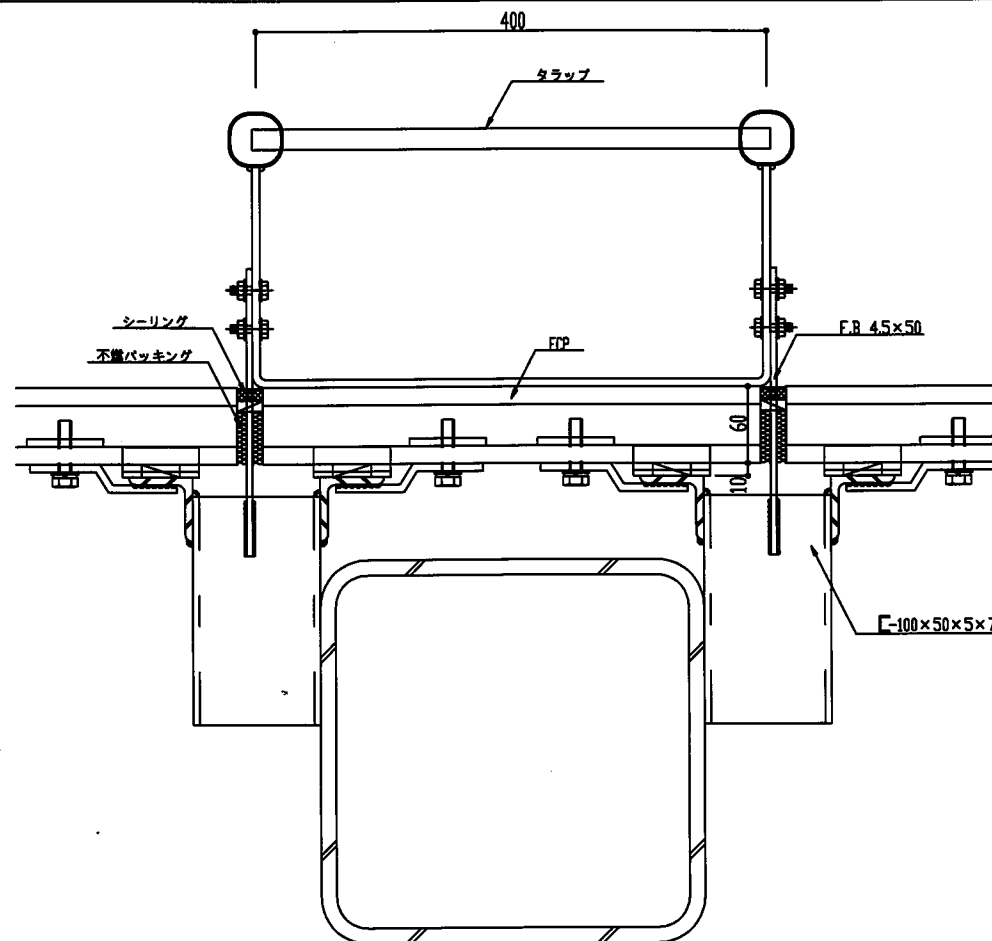
横張り工法 タラップ取合い
