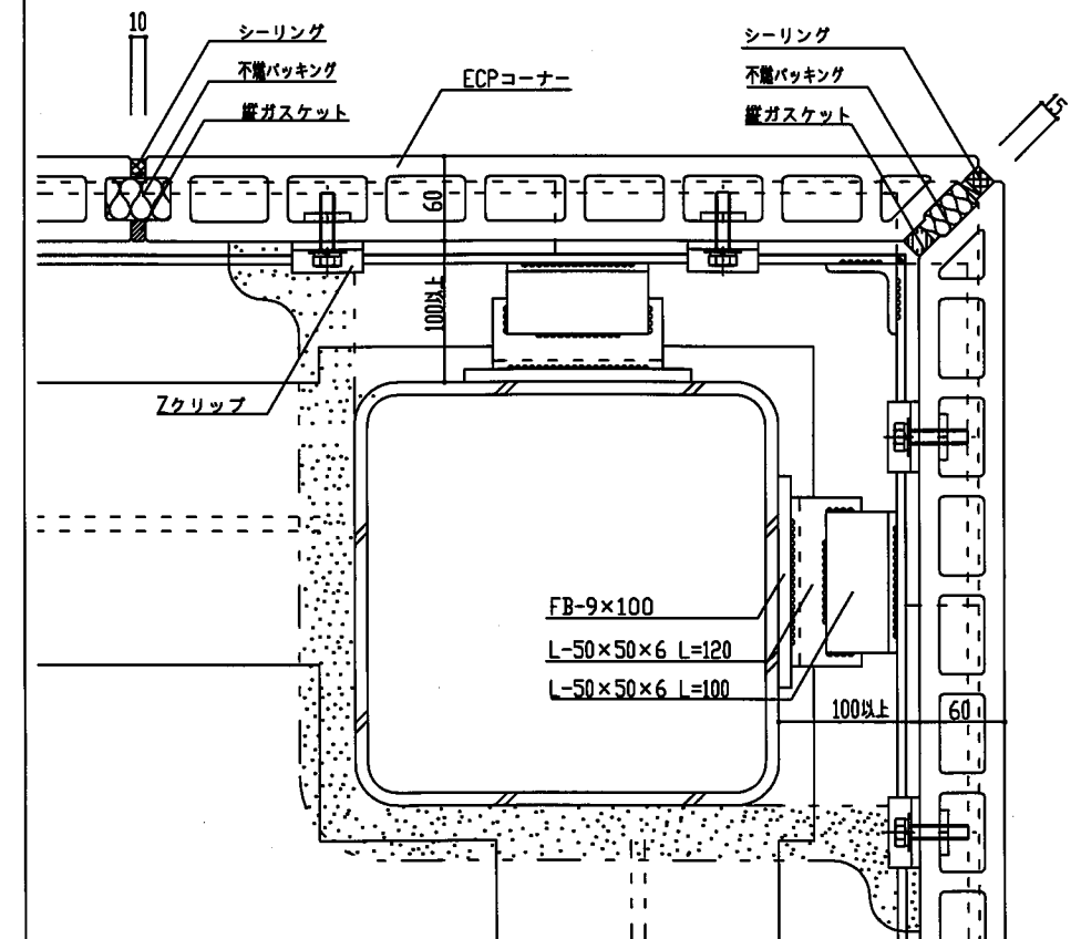
コーナー部詳細図(2)
