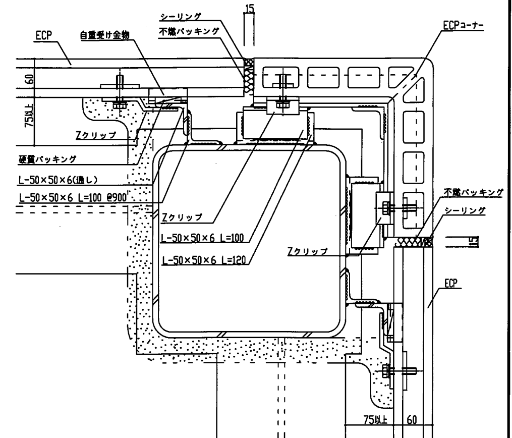
コーナー部詳細図 (1)
