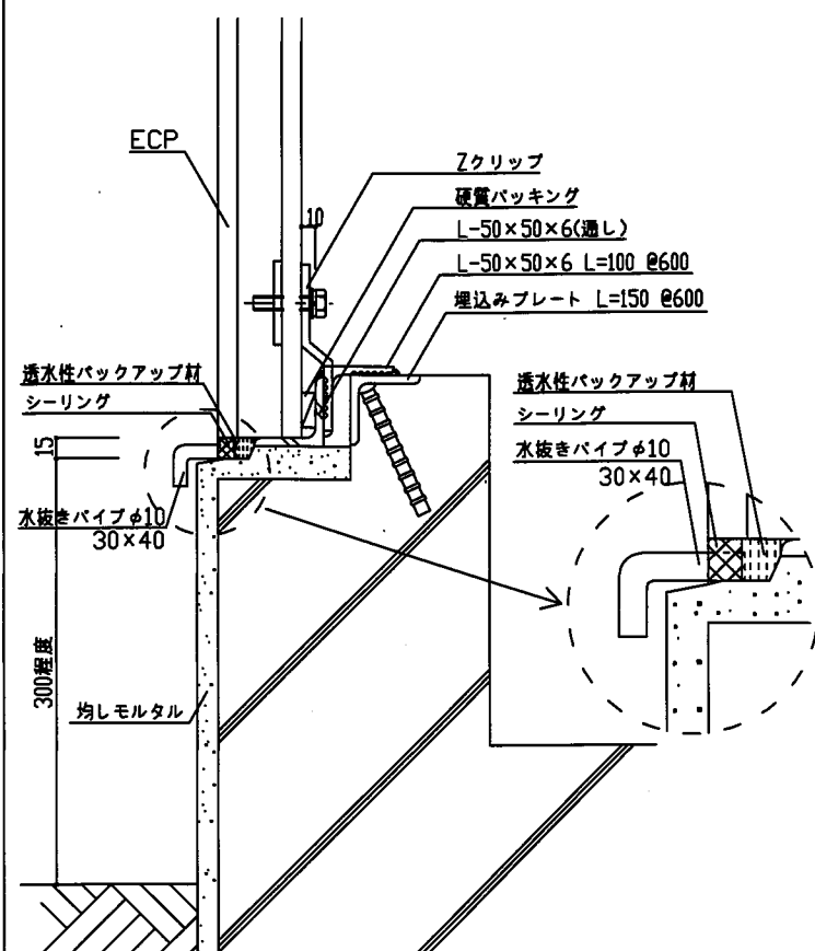
下部垂直断面詳細図
