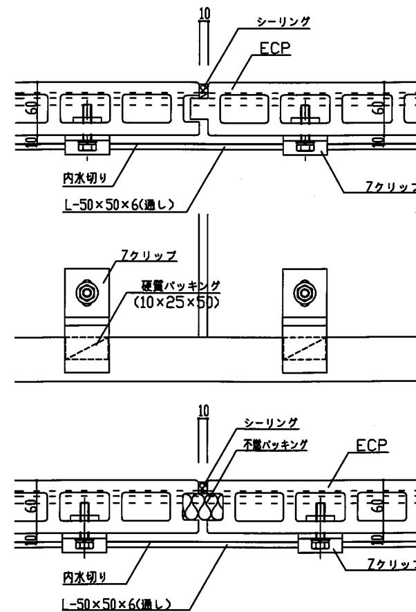
開口部垂直・水平断面詳細図
