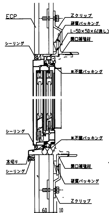
開口部垂直・水平断面詳細図
